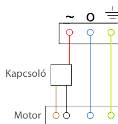
Kapcsolós motor elektromos bekötése
