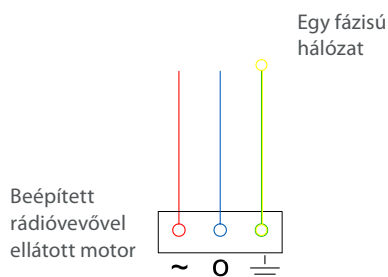
Rádiós motor elektromos bekötése
